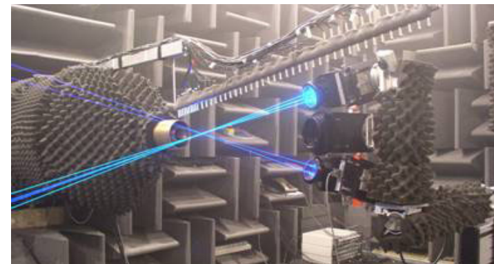
Anechoic Wind Tunnel « Bruit et Vent » © PPRIME
